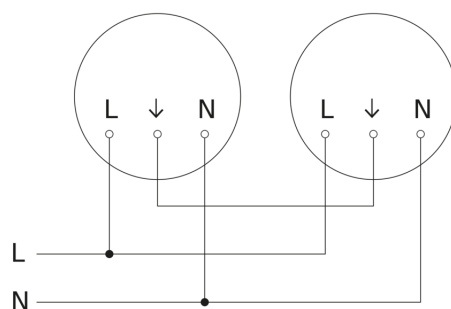
Schéma du circuit d'interconnexion maître/maître
